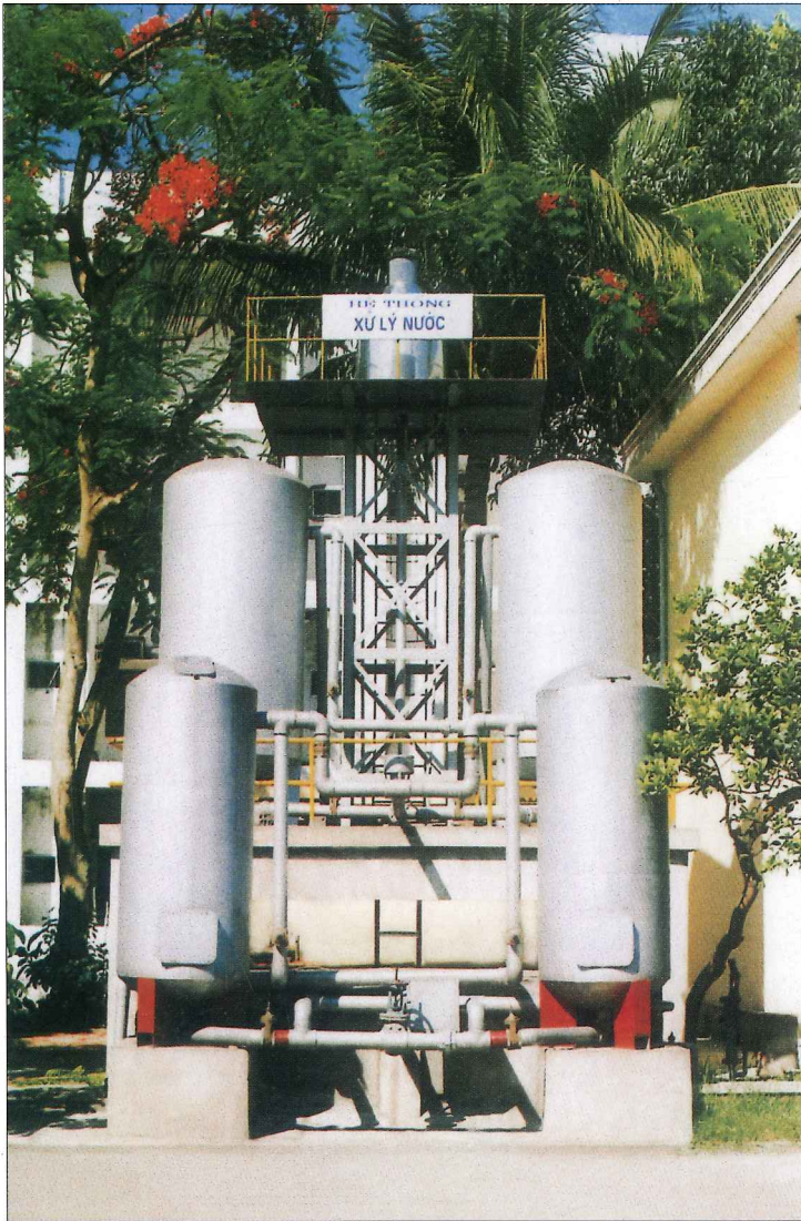
↑ Hệ thống xử lý nước tại Trung tâm phục chức năng (Cửa Lò) Bộ xây dựng Water Treatment of the rehabilitation centre ( Cua Lo) Ministry of Construction
